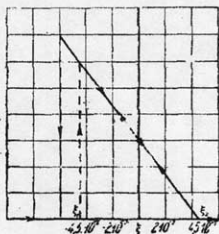
Рис. 4. Кривая гетеропараметрического резонанса ( \gamma_1 > 0 ).
