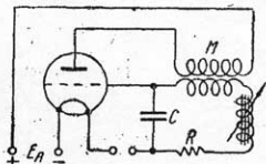
Рис. 2. Схема регенеративной системы.
