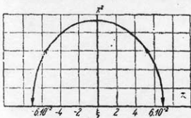
Рис. 5. Кривая гетеропараметрического резонанса в регенеративной системе (теоретическая).
