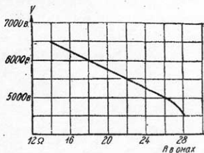
Рис. 12. Зависимость амплитуды напряжения на конденсаторе от сопротивления.
