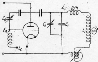
Рис. 9. Схема параметрического возбуждения в системе с регенерацией.
