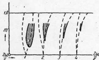
Рис. 1. Области неустойчивости (работа Андропова и Леонтовича).
