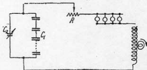
Рис. 11. Схема параметрического возбуждения в системе без регенерации.
